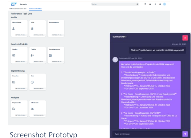
Screenshot Prototyp
